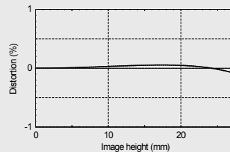
0,8m /I.S. 1:5
